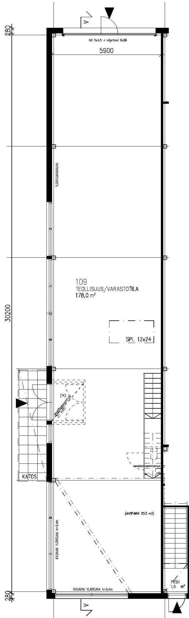
1. KERROS 1:125
